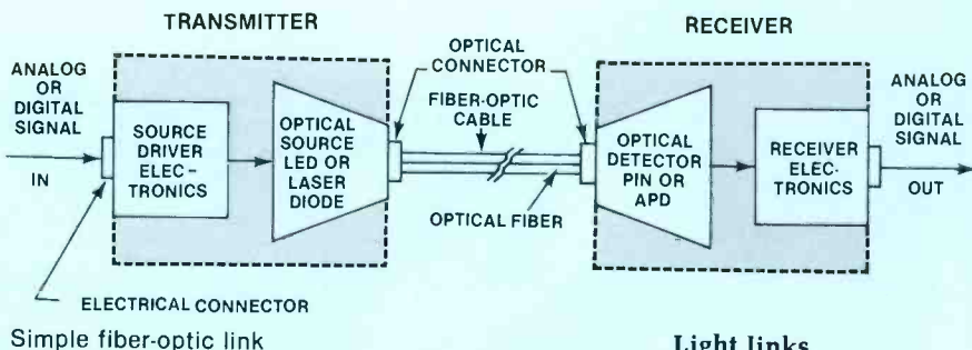
Simple fiber-optic link
